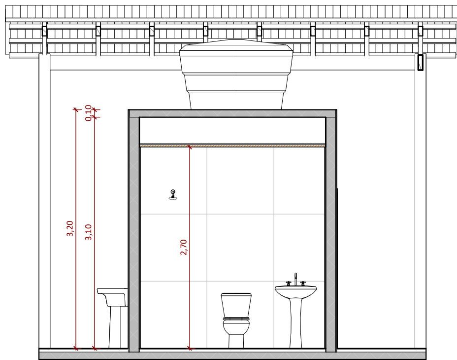
Corte 1 1 : 50
