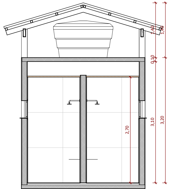
Corte 2 1 : 50
