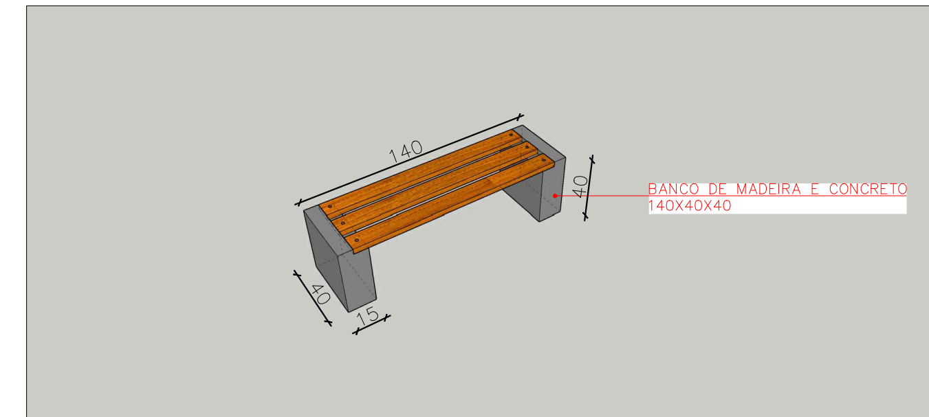
BANCO 140X40X40
