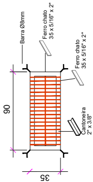
PLANTA BAIXA - TAMPA GRELHADA Sem escala
