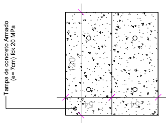
PLANTA BAIXA - TAMPA CONCRETO Sem escala
