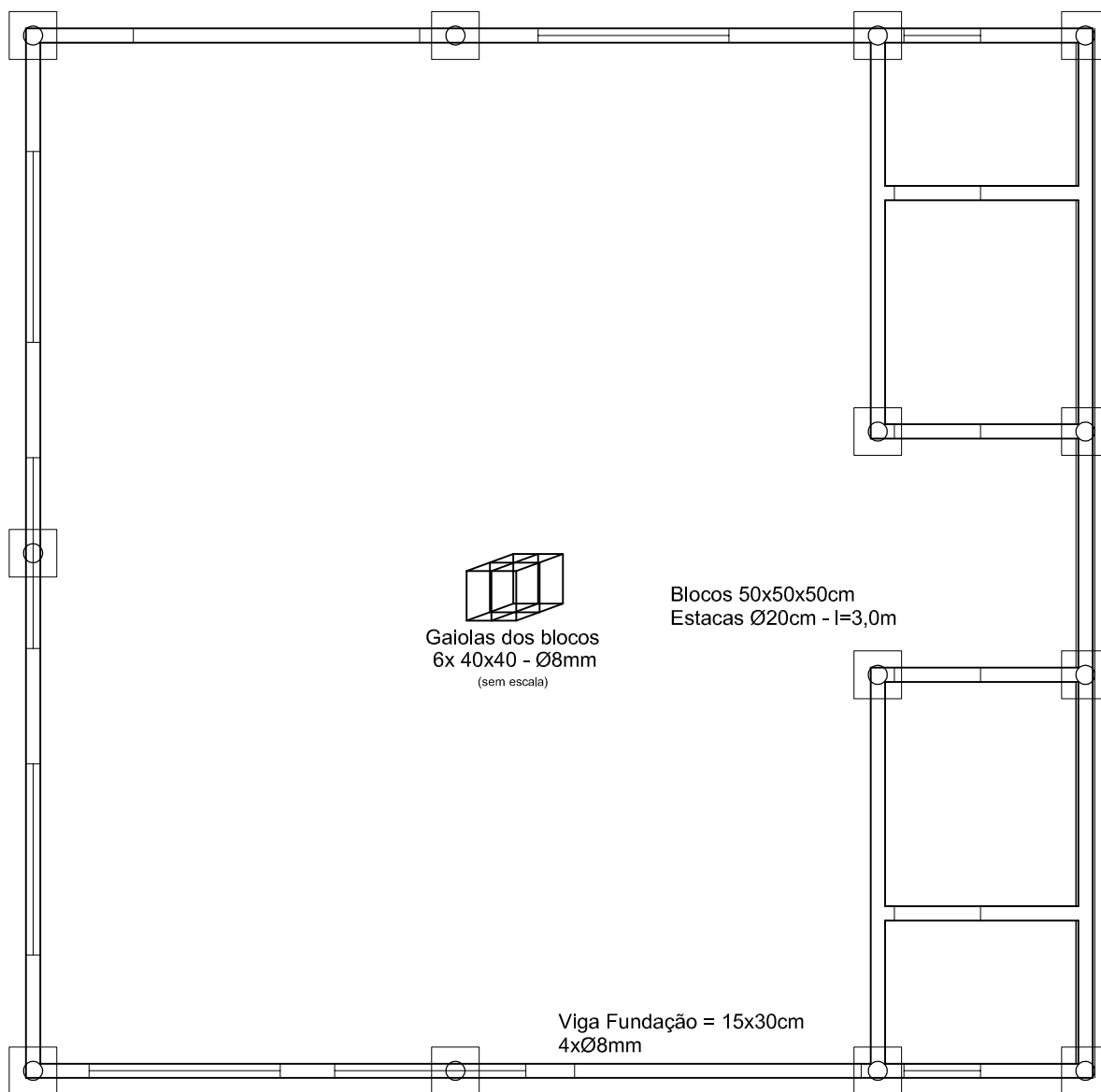
PLANTA DE FUNDAÇÕES
