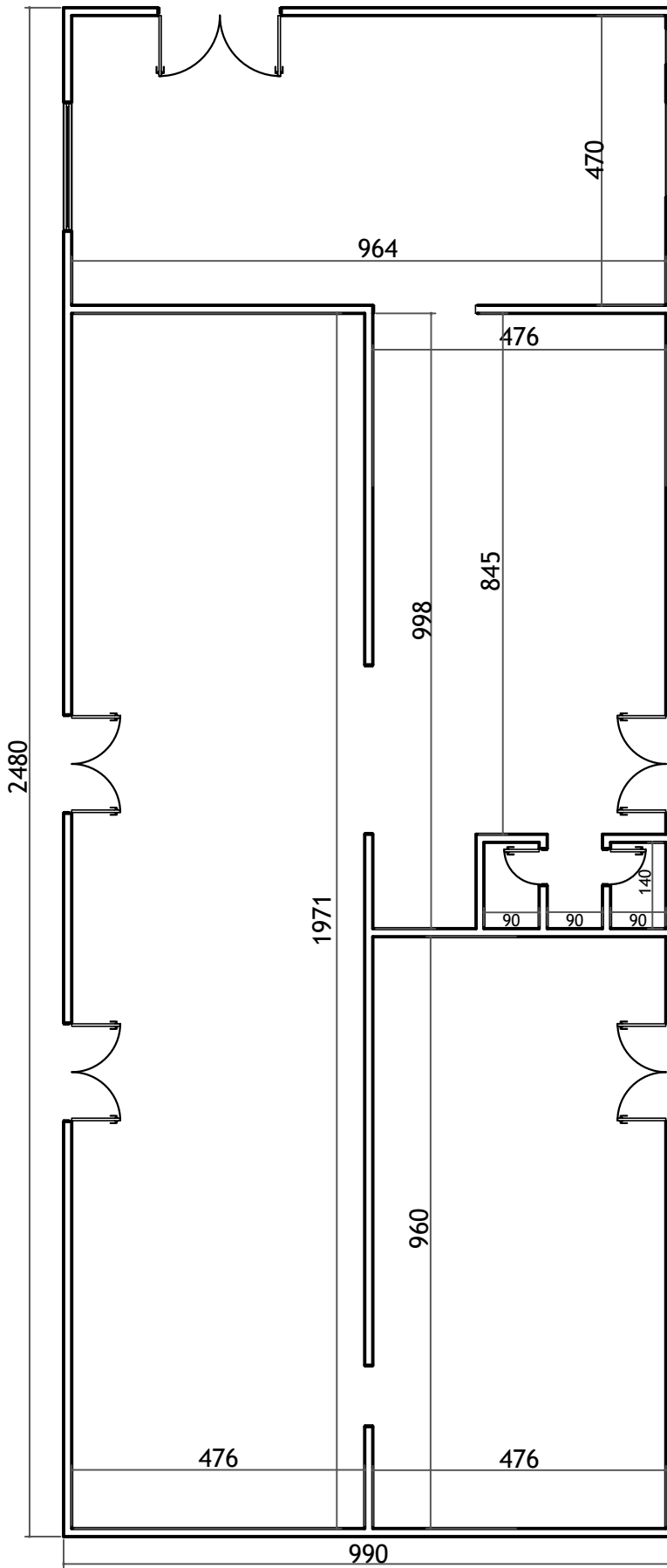
BERÇÁRIO INDUSTRIAL A=245,52m 2
