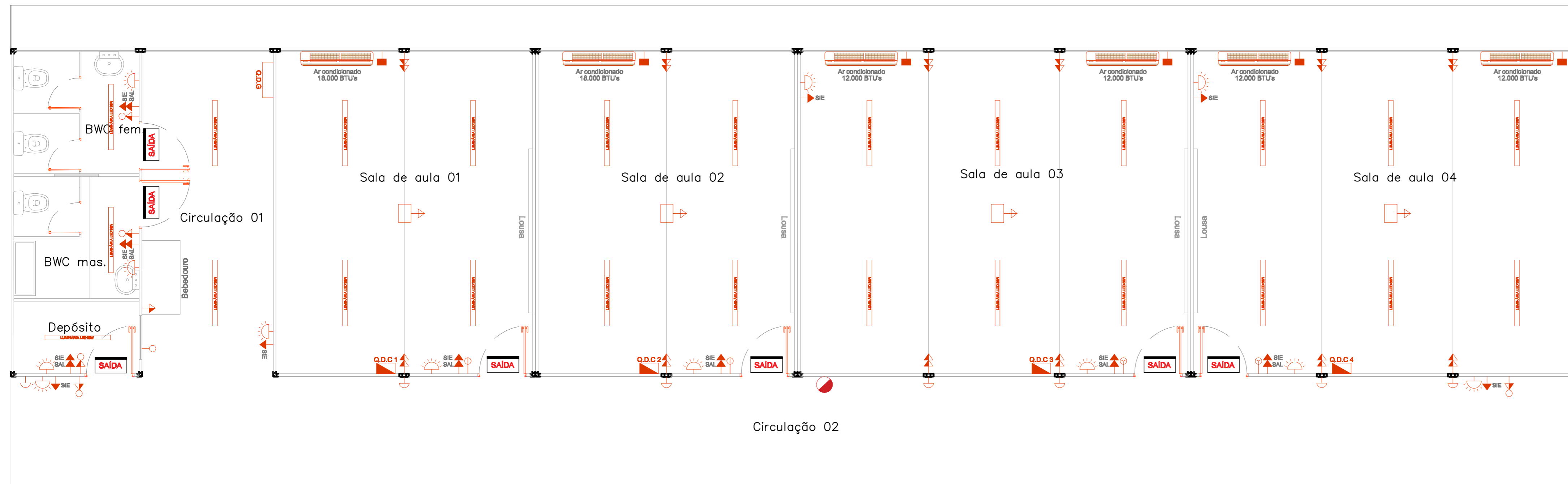
CROQUI ELÉTRICO ESC. 1:50
